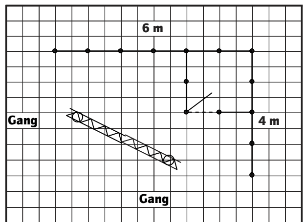
Beispiel für Eckstand 6 x 4 m Beleuchtungstraverse abgehängt
