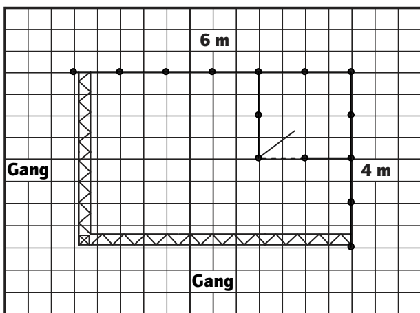
Beispiel für Eckstand 6 x 4 m Beleuchtungstraverse aufgelegt mit 1 Stütze
